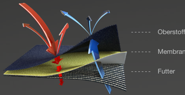
Der Twin Spacer Materialaufbau besteht aus drei Lagen: Oberstoff, Membran (GORE-TEX Fire Blocker N) und Futter (Twin Spacer)
