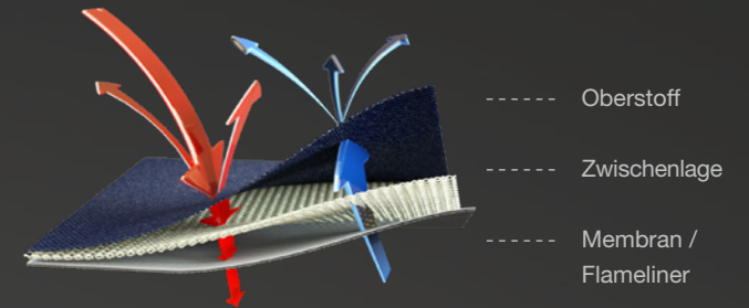
X-TREME® light besteht aus drei Lagen: Oberstoff, Zwischenlage (Heat Comfort Barrier) und Membran/Flameliner (GORE-TEX Flameliner® G und GORE-TEX Nässesperre mit GORE® CROSSTECH® Produkttechnologie)
